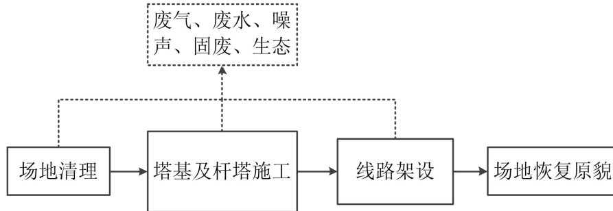
图 2 施工期工艺流程及产污环节图
