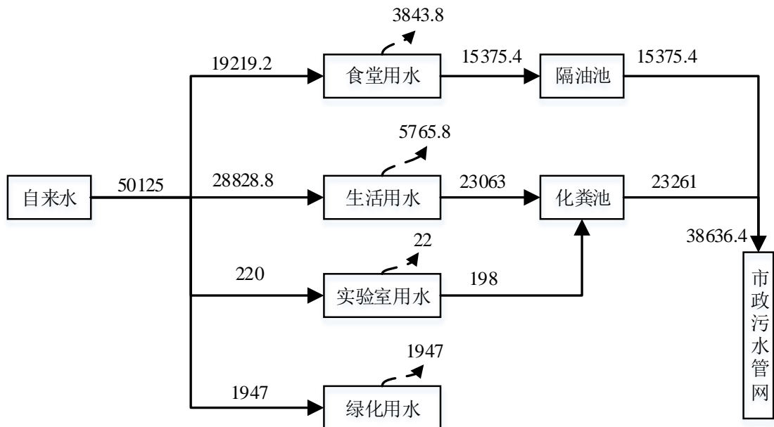
图 1 本项目水平衡图
