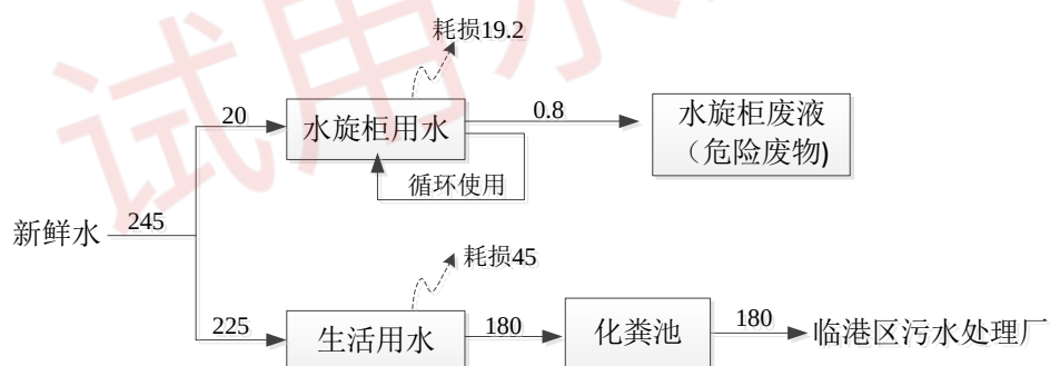
图 1-1 项目水平衡图（单位: \text{m}^3/\text{a} ）
