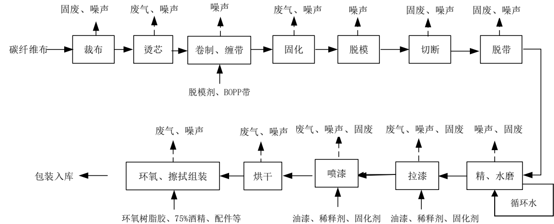
图 2-2 项目鱼竿生产工艺流程及产污环节图
