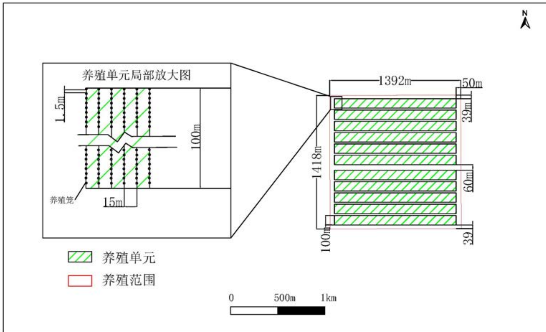
图 2.3-1 平面布置图
