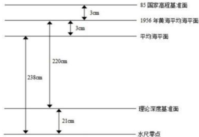
图4.12-1 基面关系图
