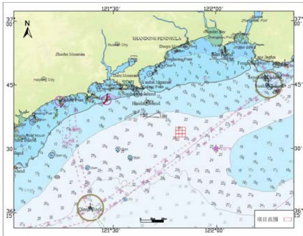
图 4.1.4-1 项目周边海域水深图
