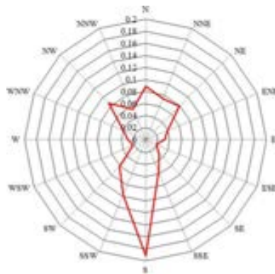
图 4.1.1-1 全年和四季代表月风向风速玫瑰图
