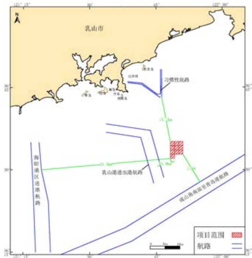
图 6.9.6-1 项目和周边航路位置关系图
