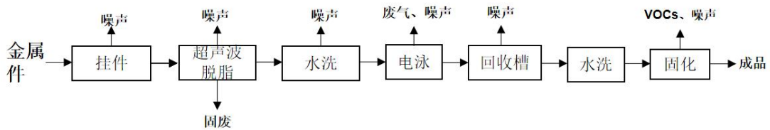
图 2-2 生产工艺流程及产污环节图
