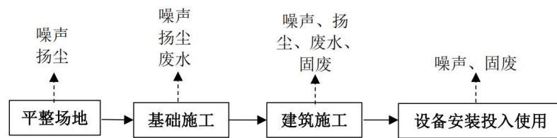
图 2-2 施工期生产工艺流程及产污环节图
