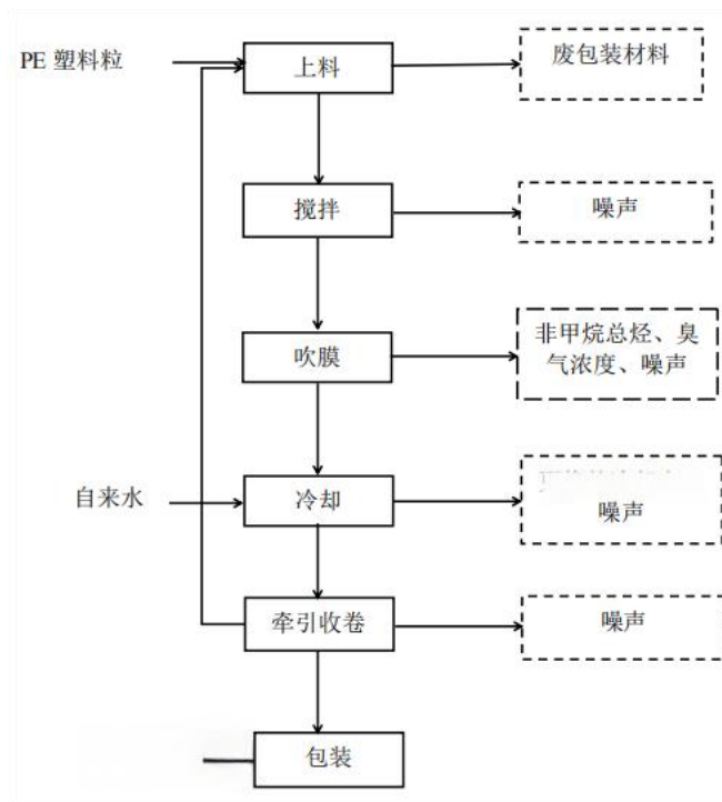
图 2-2 生产工艺流程及产污环节图
