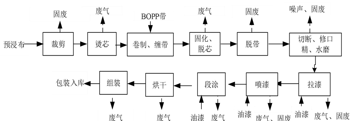
图 2-2 鱼竿生产工艺流程示意图及产污环节图
