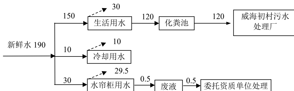
图 2-1 项目水量平衡图 (m 3 /a)
