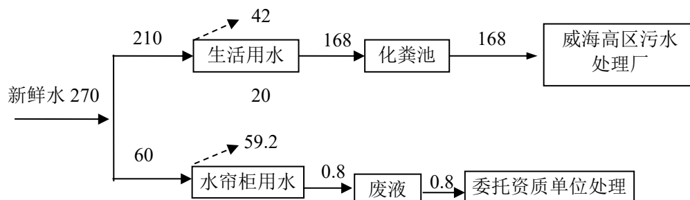
图 2-1 项目水量平衡图 ( \text{m}^3/\text{a} )
