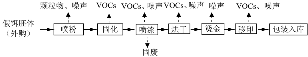
图 2-2 假饵生产工艺流程及产污环节图
