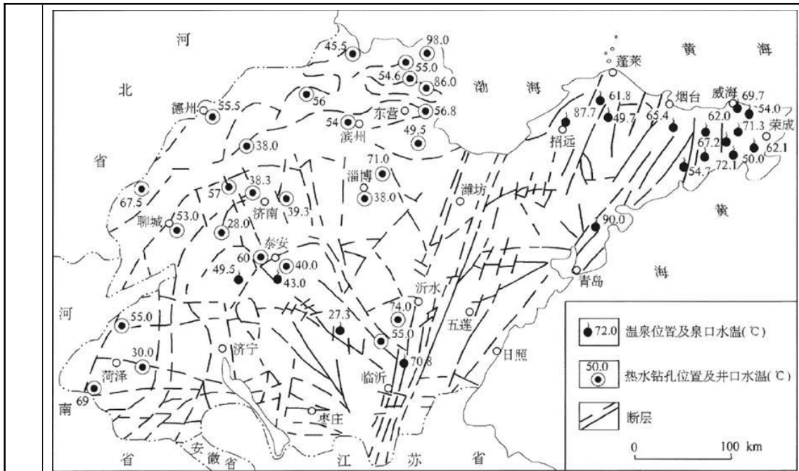
图 1.2.7-1 山东省断裂构造图
