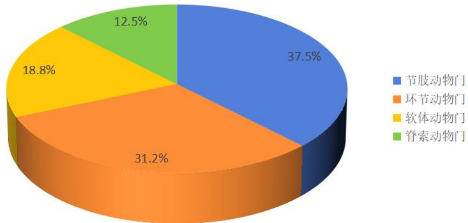
图 1.2.9.4-6 大型底栖生物种类组成
