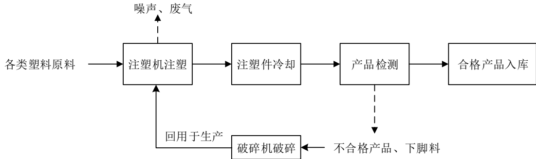
图 2-2 项目塑料制品生产工艺流程图及产污环节图
