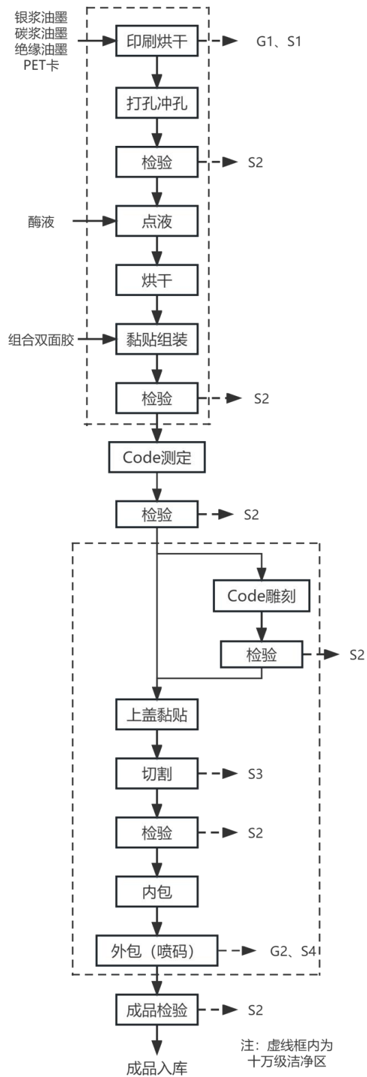
图 2.2 血糖试纸条工艺流程及产污环节
