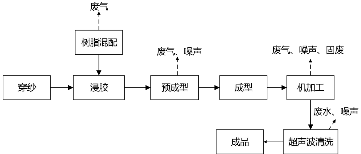
图 2-1 运营期生产工艺流程及产污环节图
