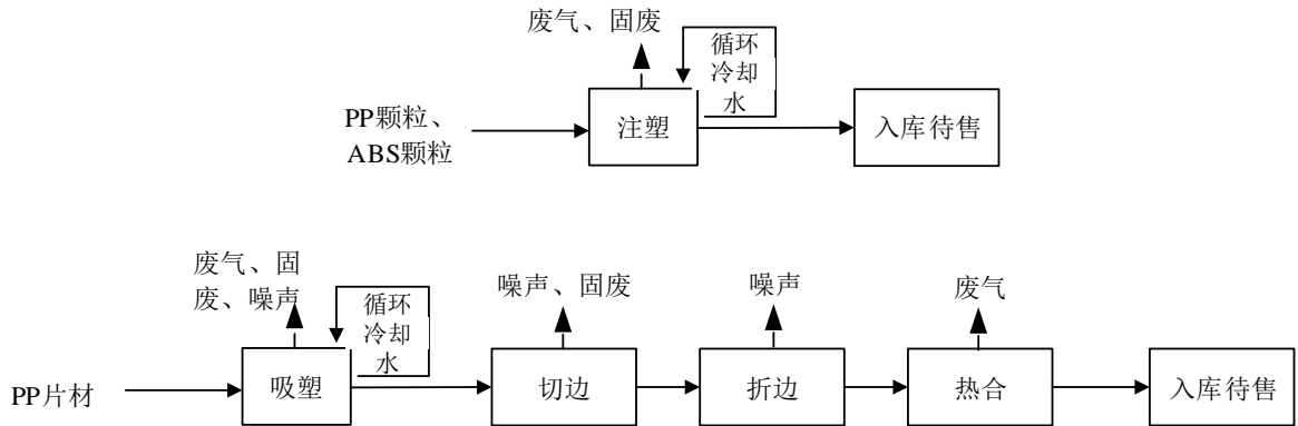
图 2-1 项目生产工艺流程图及产污环节图
