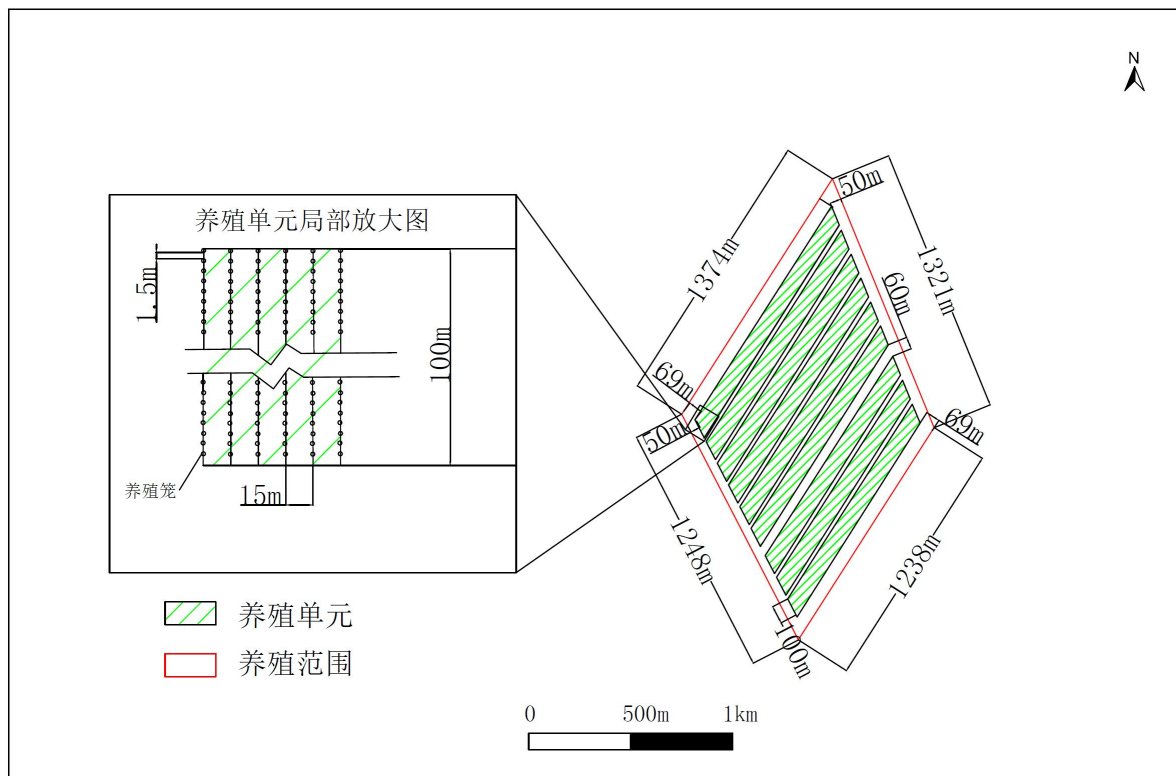
图 2.3-1b 平面布置（养殖区 1）
