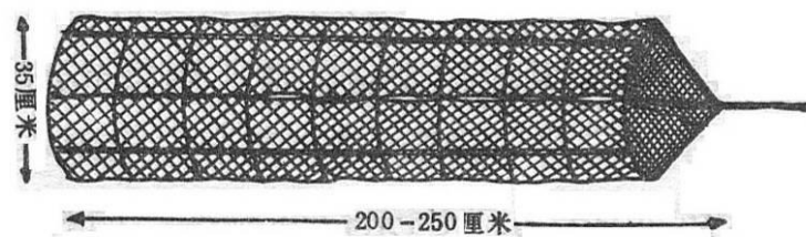
图 2.3-3 挂籠結構圖
