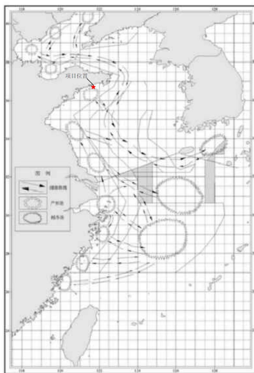
银鲳鱼洄游分布示意图
