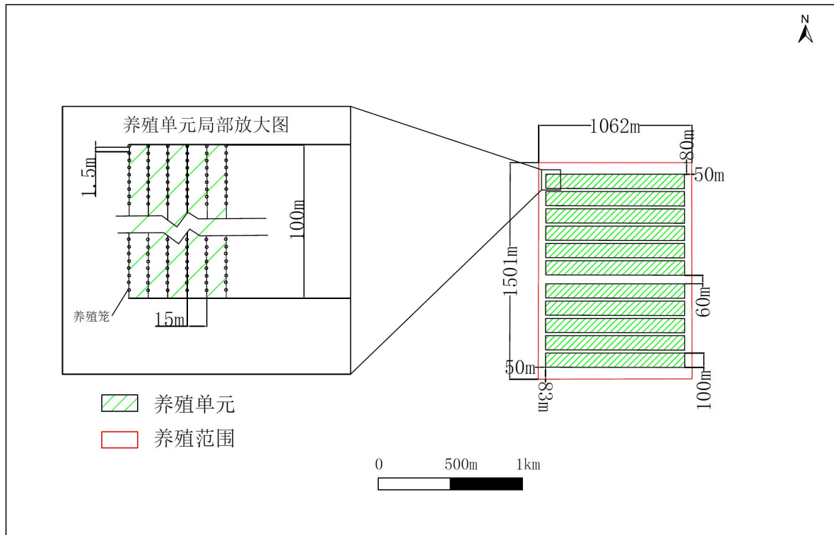
图 2.3-1b 平面布置（养殖区 8）
