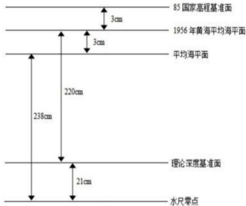
图4.12-1 基面关系图
