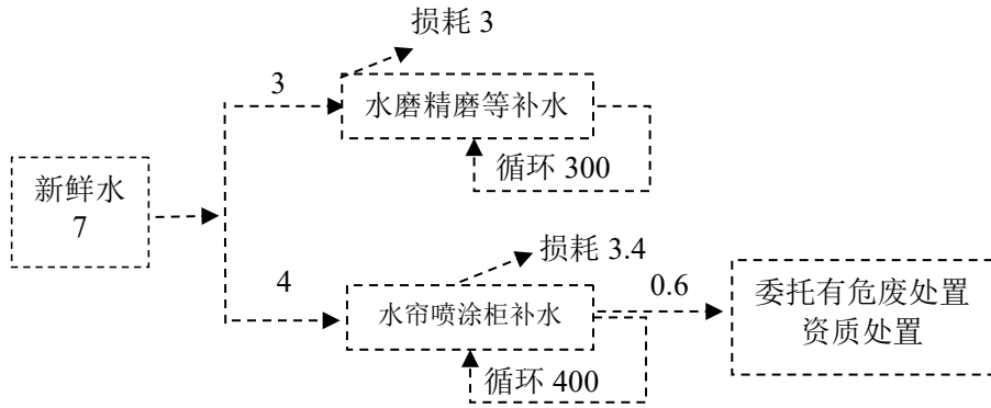
图 2-1 项目水量平衡图 (t/a)
