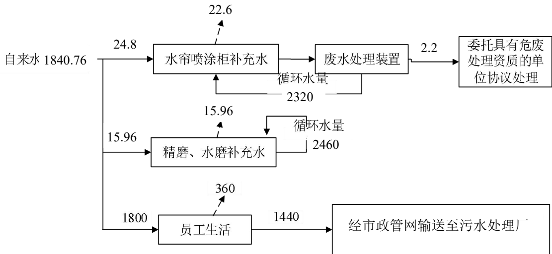
图 2-2 全厂水平衡图 (t/a)
