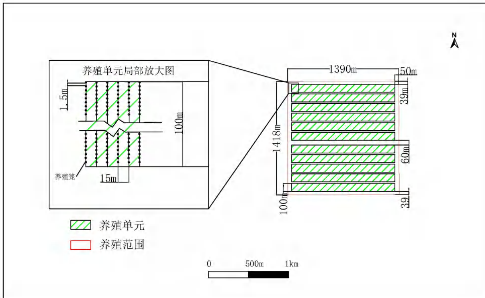
(c) 代表性养殖单元平面布置示意 (单元4)
