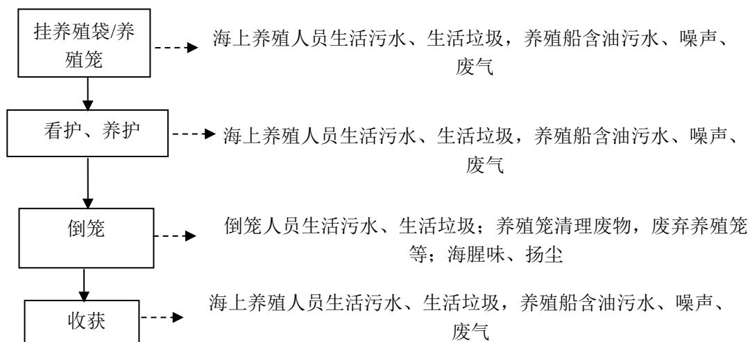
图 3.1.1-2 运营工艺及产污环节示意图
