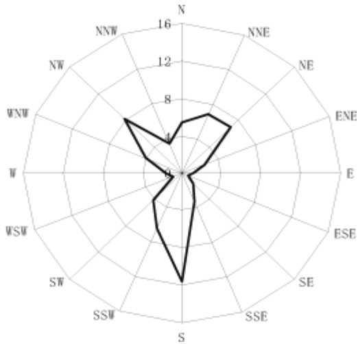
图 4.1.2-2 累年各向风浪频率玫瑰图
