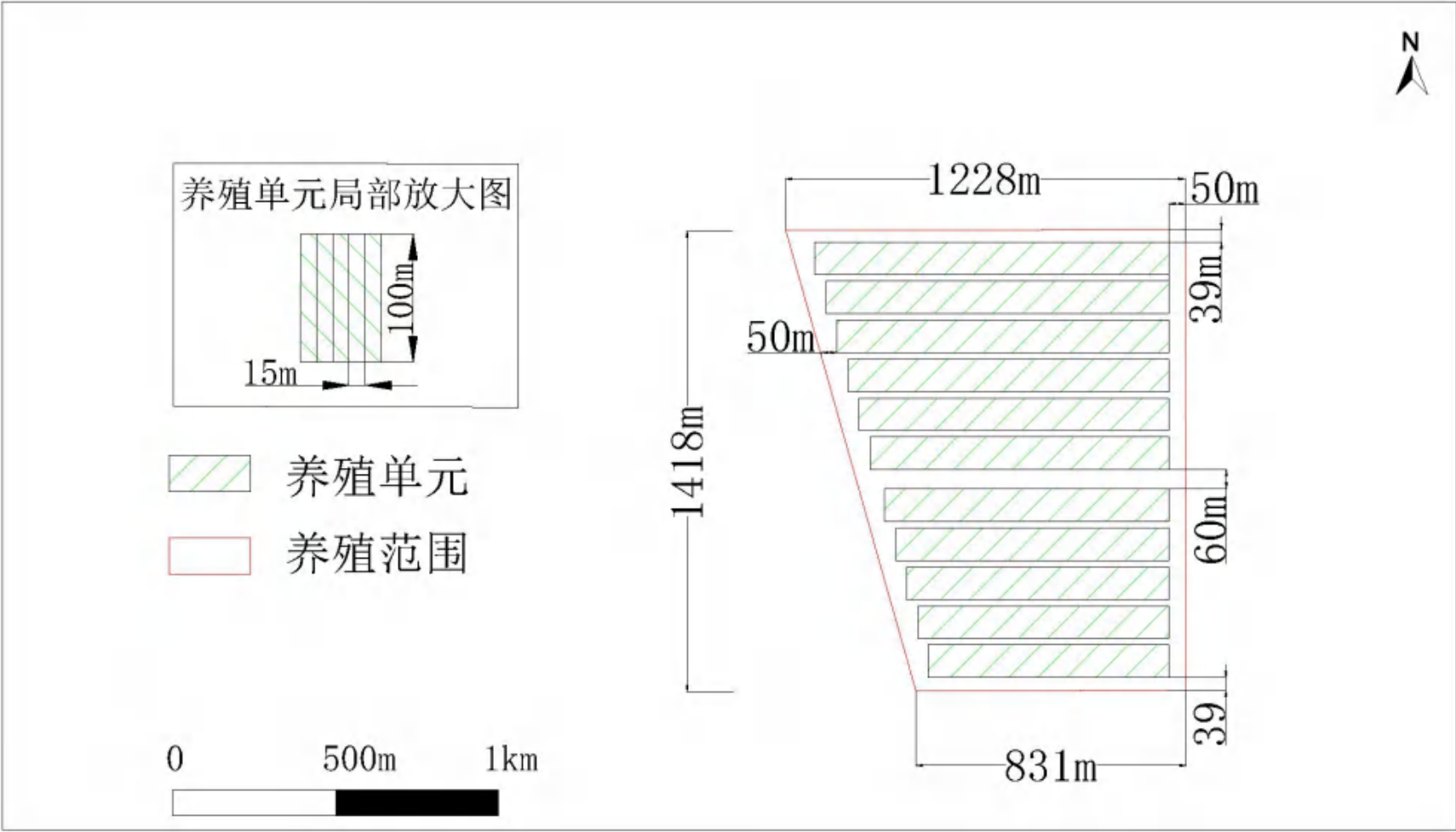
(h) 代表性养殖单元平面布置示意 (单元 22)
