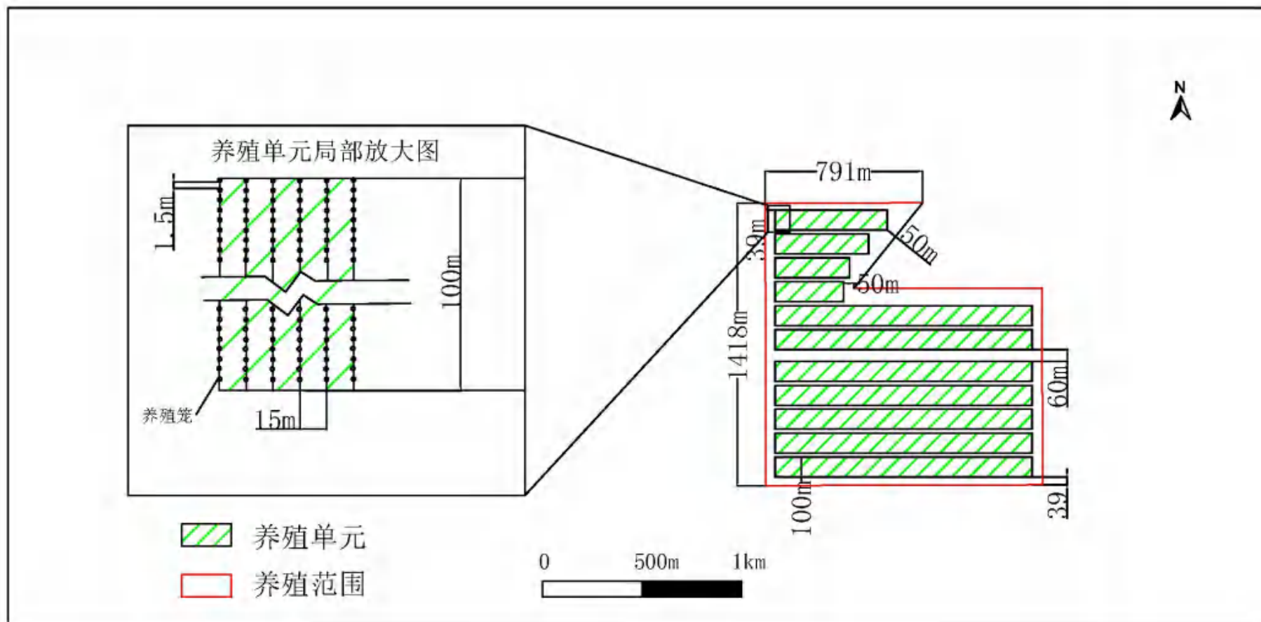
(d) 代表性养殖单元平面布置示意 (单元 5)
