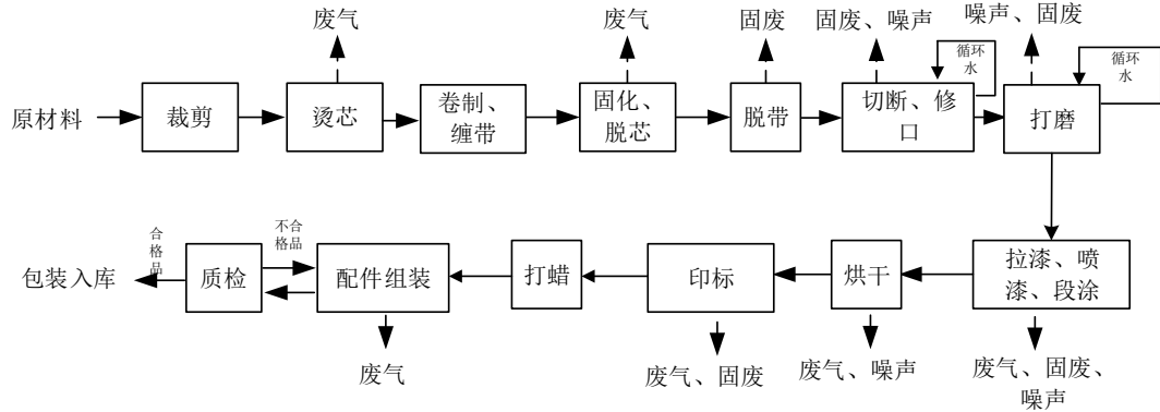
图 2-1 项目生产工艺流程图及产污环节图
