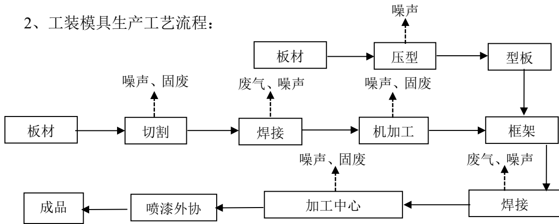
图 2-1 工装模具生产工艺流程及产污环节图
