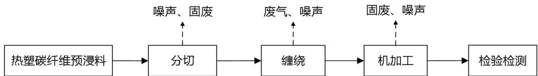
图 2-1 新能源储能产品生产工艺流程及产污环节图
