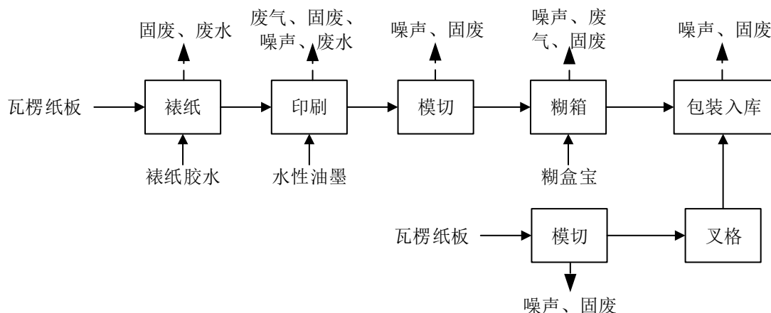
图 2-1 项目生产工艺流程示意图及产污环节图
