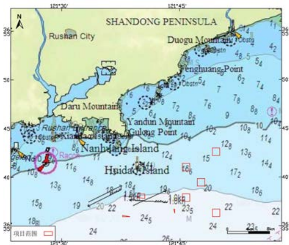
图 4.1.4-1 项目周边海域水深图
