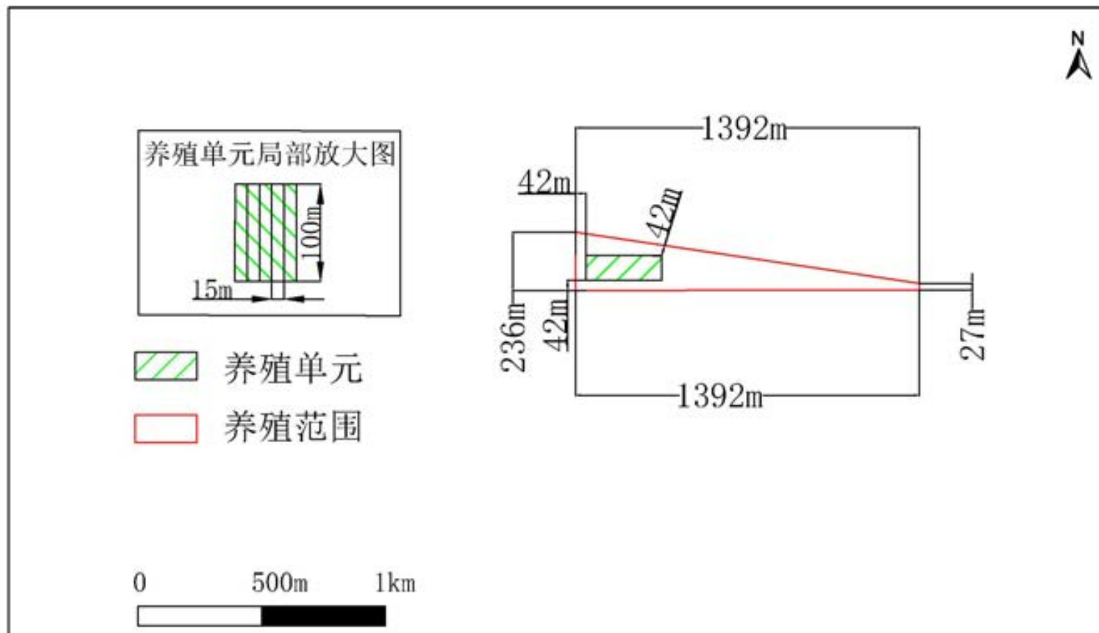
(d) 代表性养殖单元平面布置示意 (单元 6)
