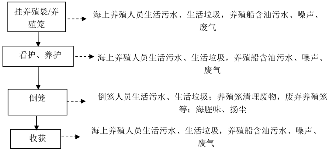
图 3.1.2-1 运营工艺及产污环节示意图
