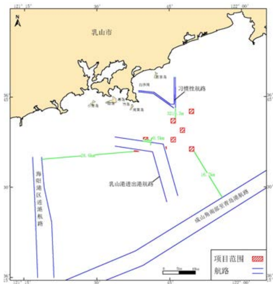
图 6.9.6-1 项目和周边航路位置关系图
