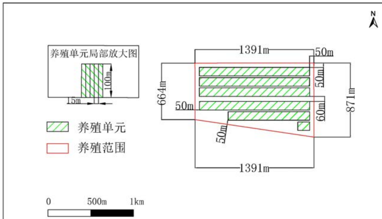
(c) 代表性养殖单元平面布置示意 (单元4)
