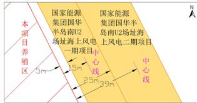
图 6.9.5-1 养殖区与电缆管道的位置关系放大图
