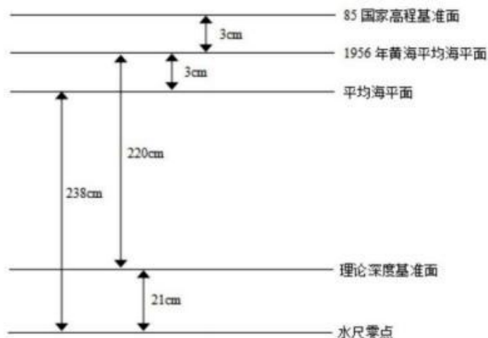
图4.1.2-1 基面关系图
