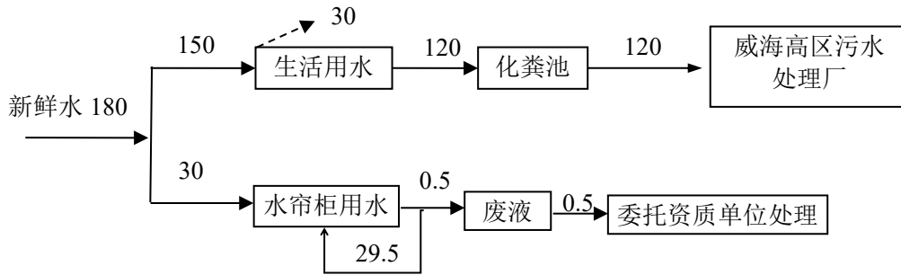
图 2-1 项目水量平衡图 (m 3 /a)
