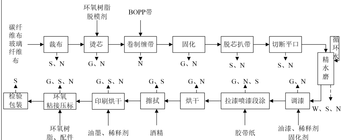
图 2-2 项目生产工艺流程及产污环节图
