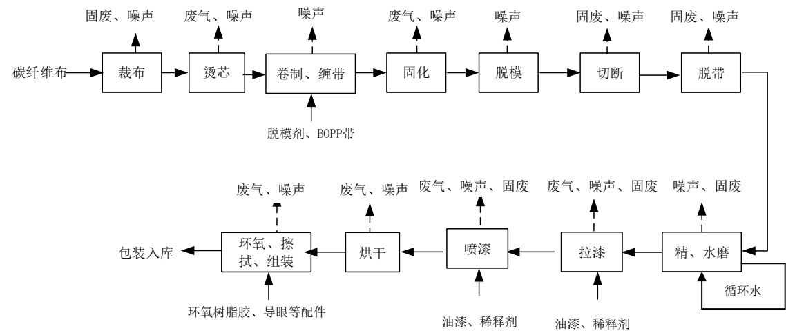
图 2-2 项目鱼竿生产工艺流程及产污环节图
