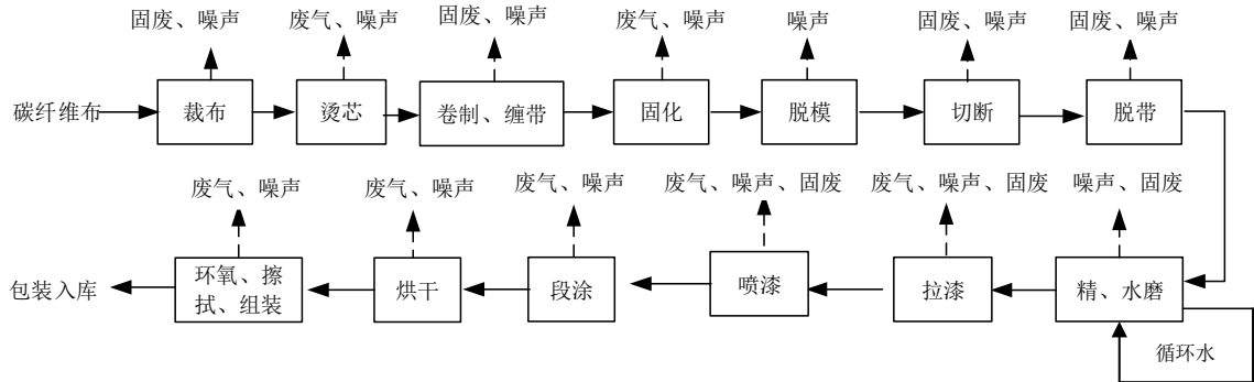
图 2-2 项目鱼竿生产工艺流程及产污环节图
