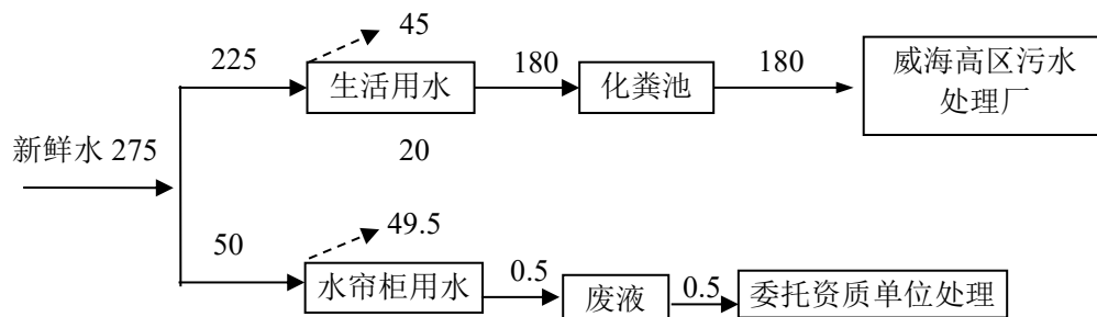
图 2-1 项目水量平衡图 (m 3 /a)
