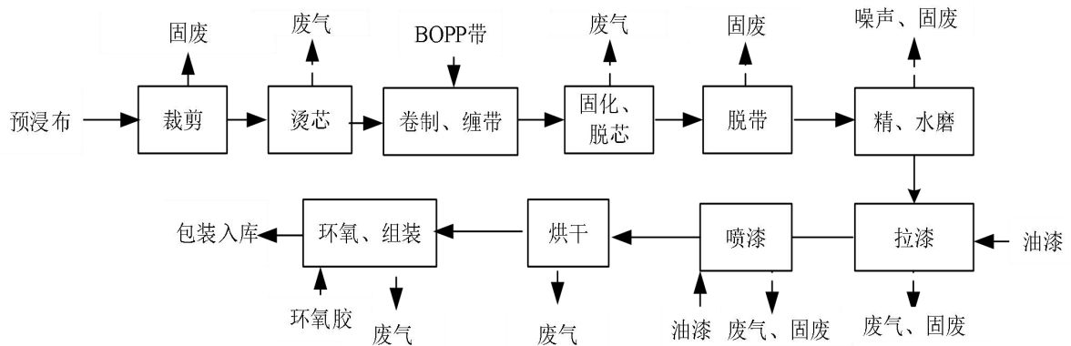
图 2-2 鱼竿生产工艺流程示意图及产污环节图
