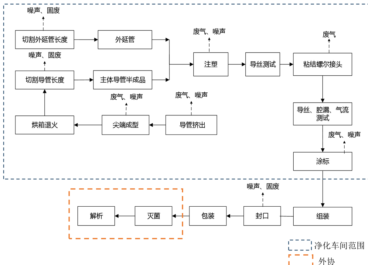
图 2-1 运营期生产工艺流程及产污环节图
