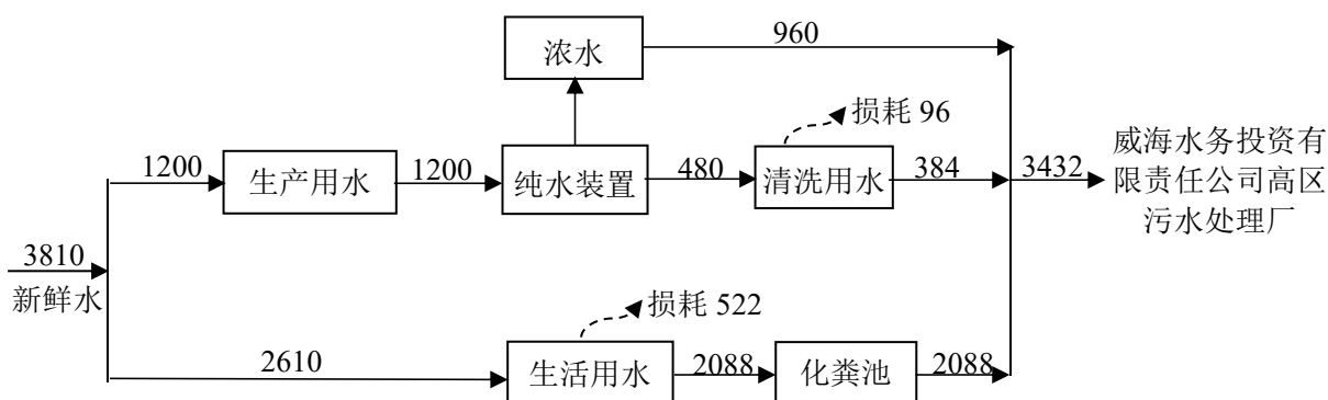
图 2-1 项目水平衡图 (单位: \text{m}^3/\text{a} )
