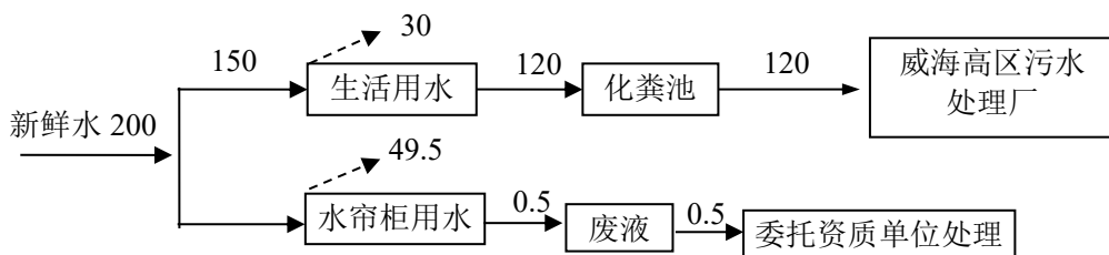
图 2-1 项目水量平衡图 ( \text{m}^3/\text{a} )
