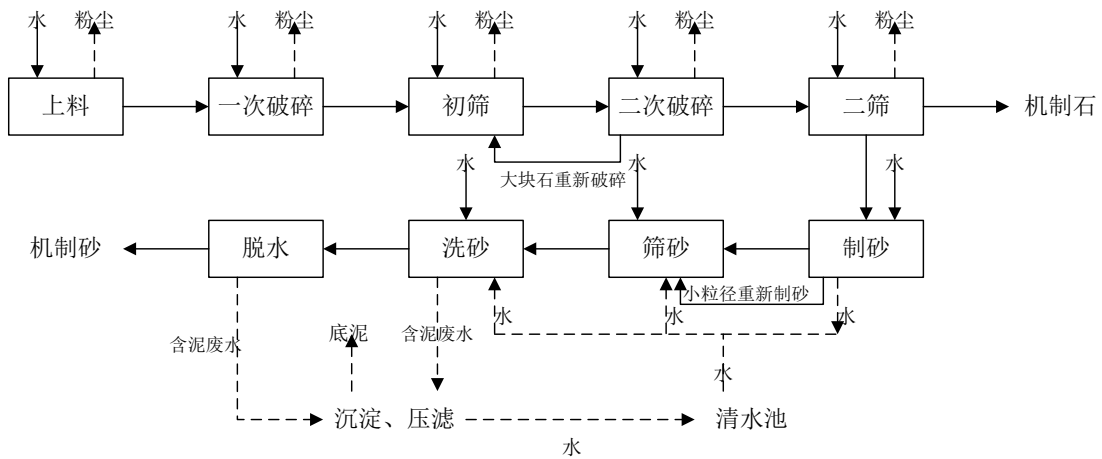
图 2-2 机制砂石工艺流程图及产污环节图
