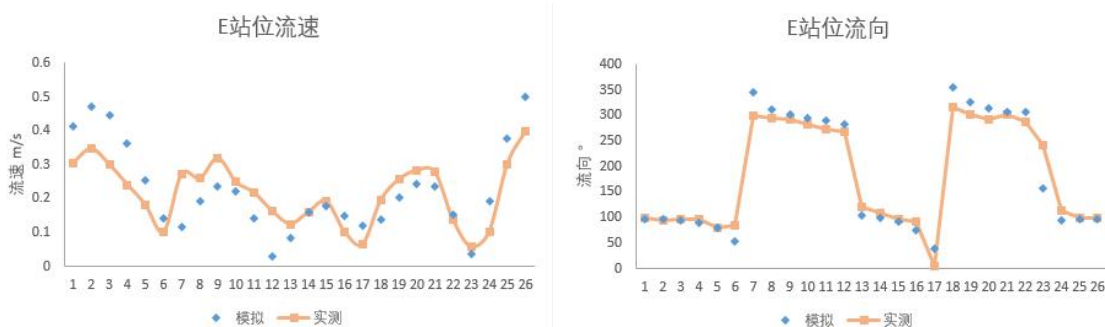
图 4.2-6e E 站位潮流流速、流向验证曲线
