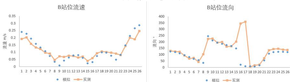
图 4.2-6b B 站位潮流流速、流向验证曲线
