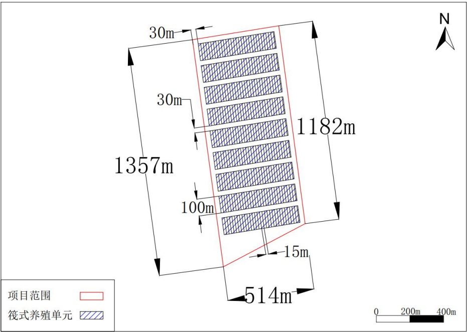
图 2-3b 项目总平面布置图（筏式养殖区）
