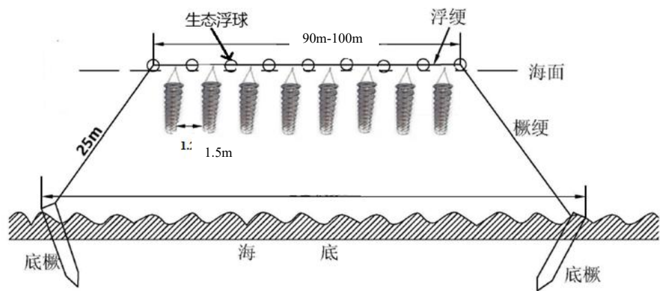
图 2-4 浮纜、橈纜、浮漂和挂笼结构图
