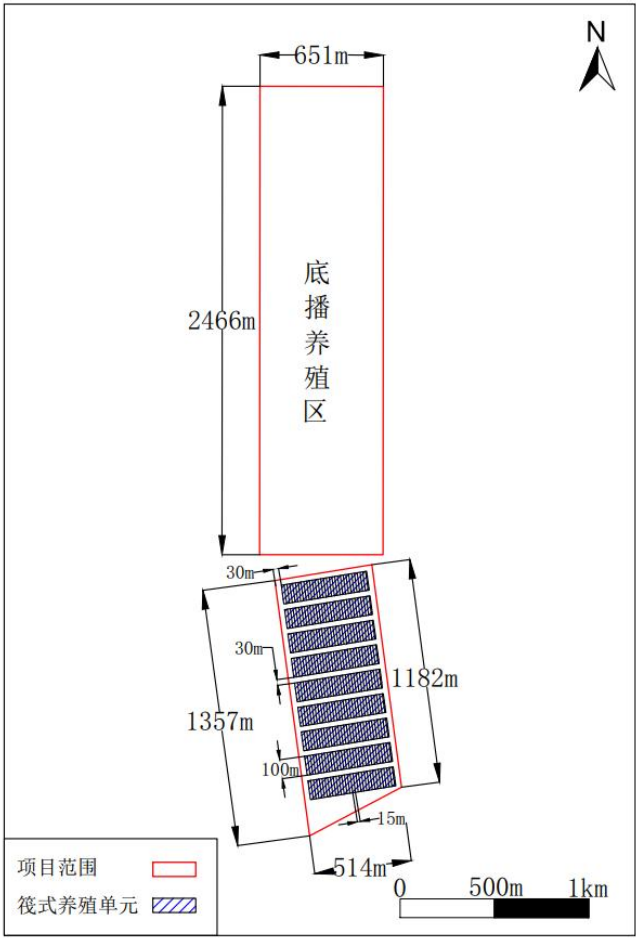
图 2-3a 项目总平面布置图
