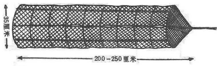
图 2-5 挂笼结构图
