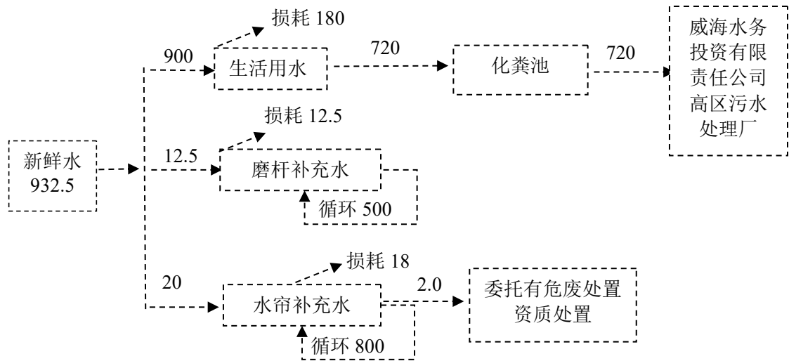
图 2-1 项目水量平衡图 (t/a)
