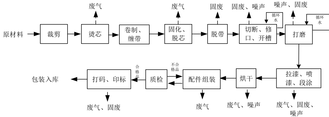
图 2-1 项目生产工艺流程示意图及产污环节图
