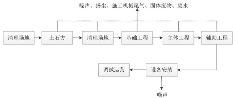
图 2-9 施工流程及产污环节图
