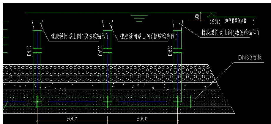
图 2-5 海水淡化管路排水口结构图
