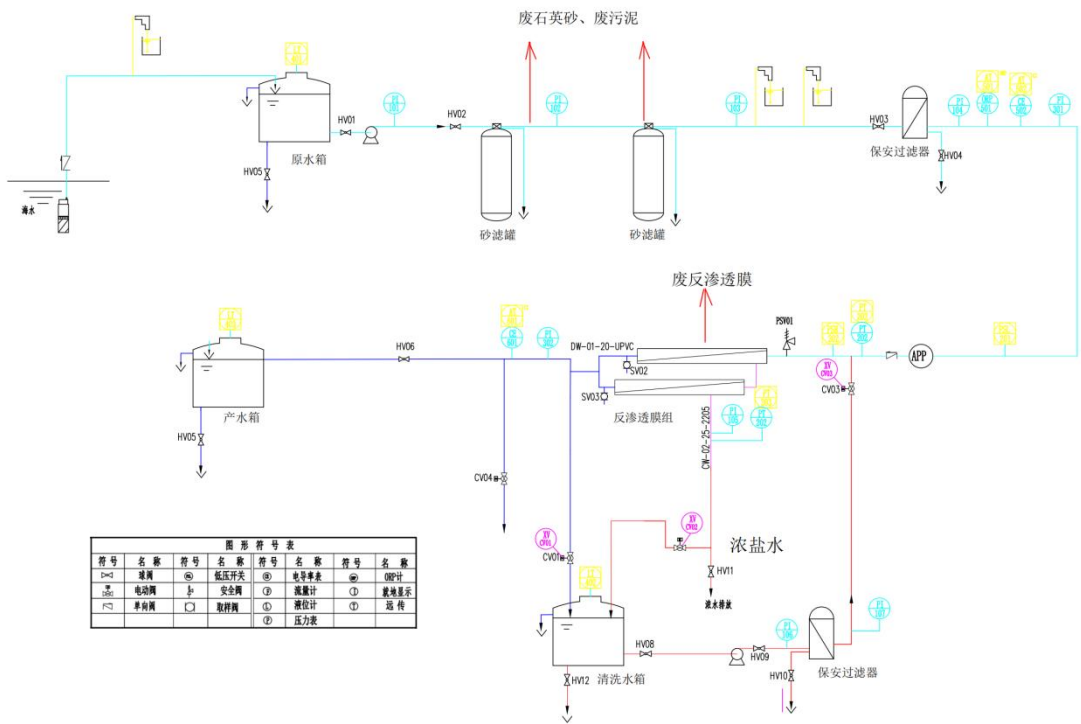
图 2-10 海水淡化工艺流程及产污环节
