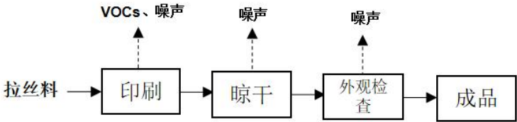
图 2-1 生产工艺流程及产污环节图
