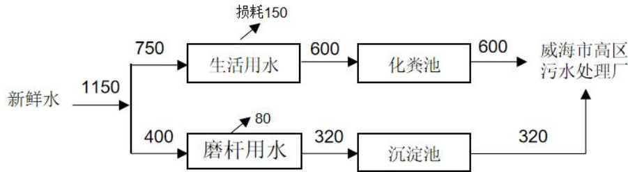
图 2-1 项目水量平衡图 (m 3 /a)
