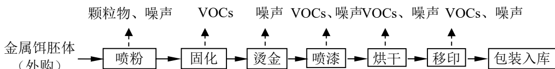
图 2-2 金属饵生产工艺流程及产污环节图
