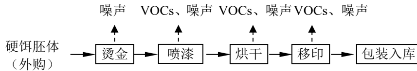
图 2-3 硬饵生产工艺流程及产排污环节图
