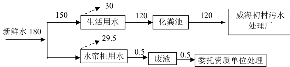
图 2-1 项目水量平衡图 (m 3 /a)
