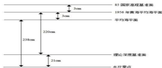
图4.1.2-1 基面关系图
