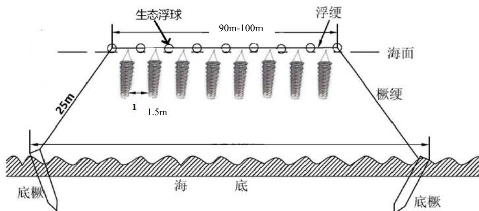
图 2-4 浮纜、概纜、浮漂和挂笼结构图
