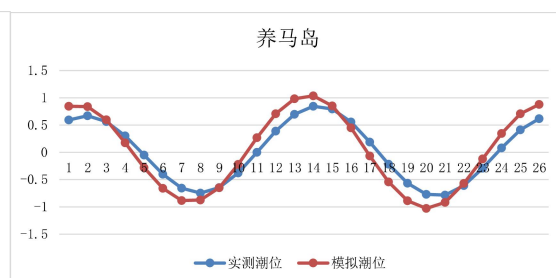
图 4.2-5b 潮位验证曲线（养马岛）
