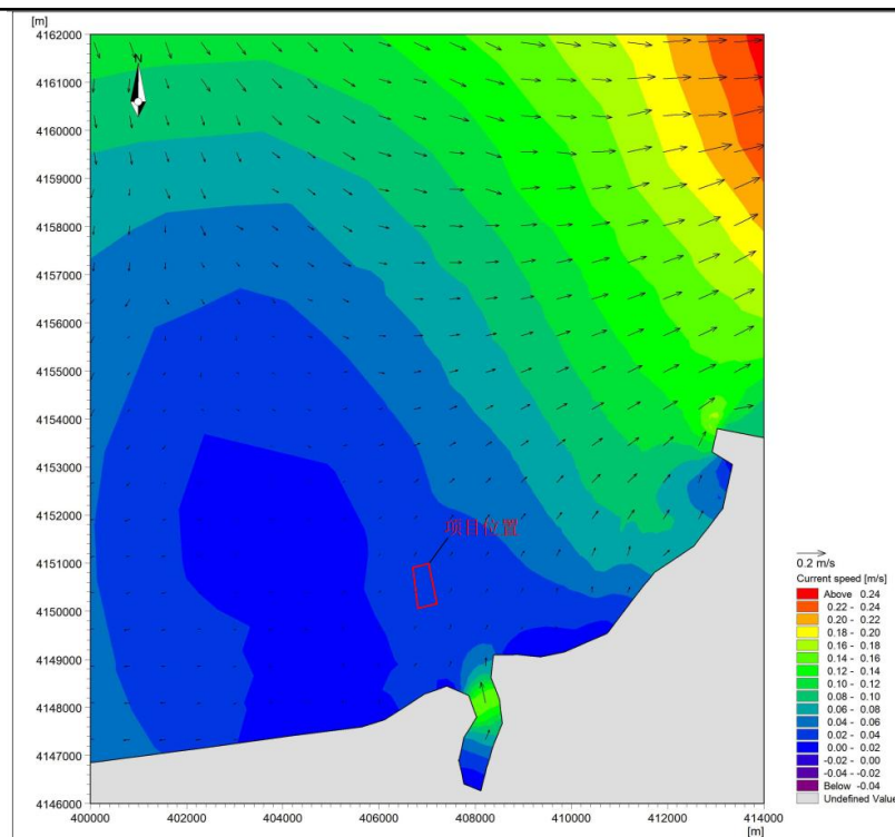
图 4.2-8 工程附近海域潮流场（落急）
