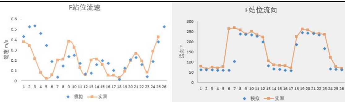
图 4.2-6f F 站位潮流流速、流向验证曲线
