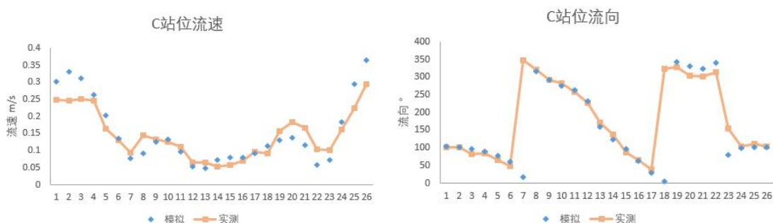
图 4.2-6c C 站位潮流流速、流向验证曲线
