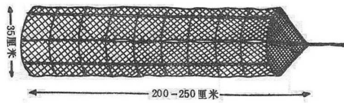
图 2-5 挂笼结构图
