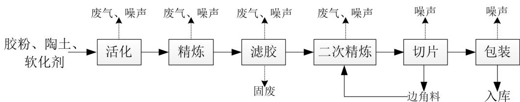
图 2-2 项目生产工艺流程及产污环节图
